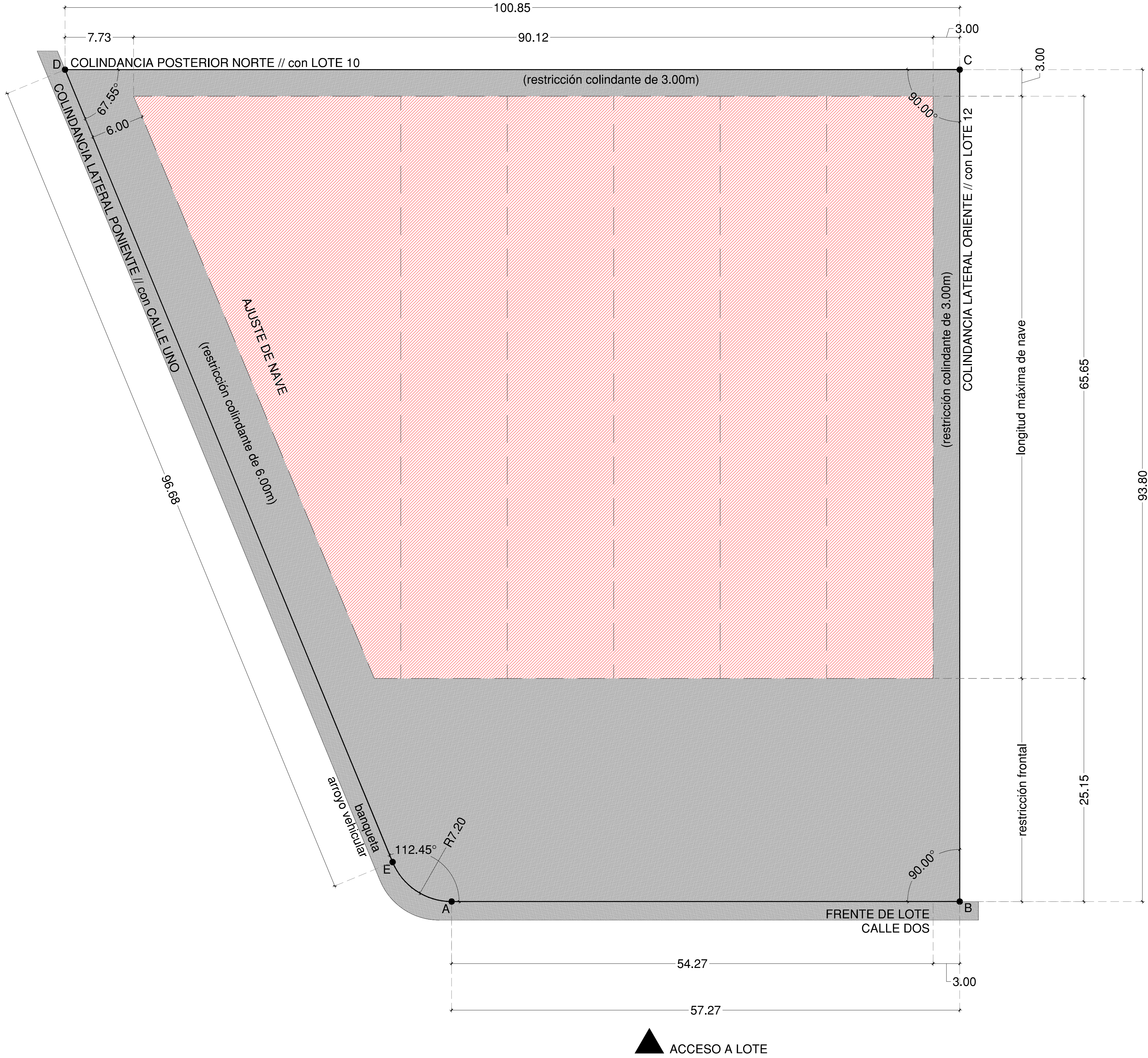
PLANTA > LOTE 11 PIA // PARQUE INDUSTRIAL AEROPUERTO, QRO.-MX
